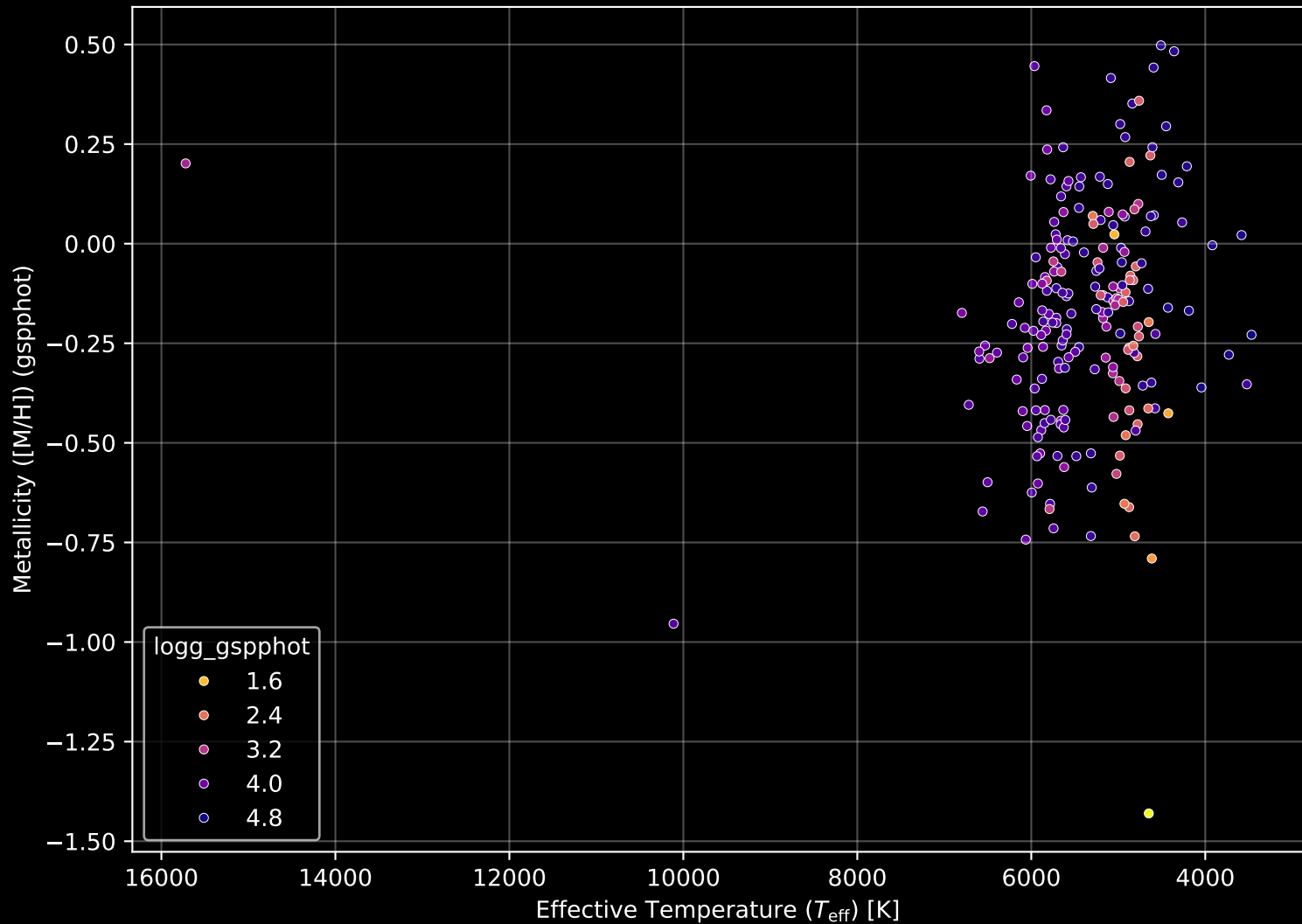
APOGEE DR17 Field: [271-36-O_TESS] Stellar Population Parameters (n= 208)
